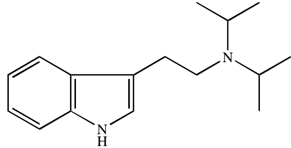
25 N,N-ジイソプロピルトリプタミン及びその塩類 N,N-diisopropyltryptamine DIPT
