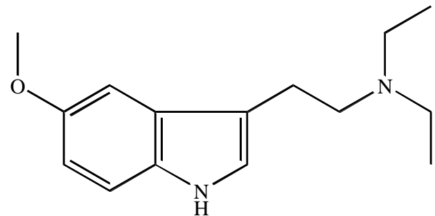
26 N,N-ジエチル-5-メキソトリプタミン及びその塩類 N,N-diethyl-5-methoxytryptamine 5-MeO-DET
